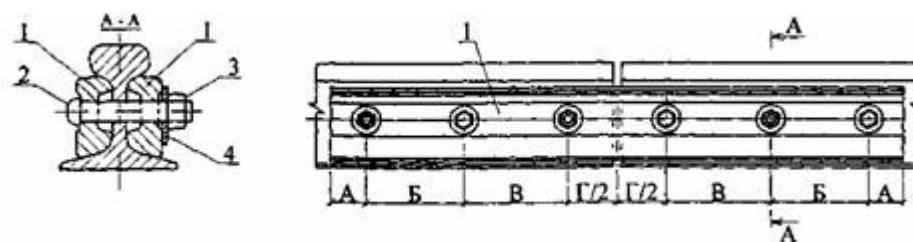
Рис. П.7.2. Стыковое разъемное крепление для направляющих типа Р.
