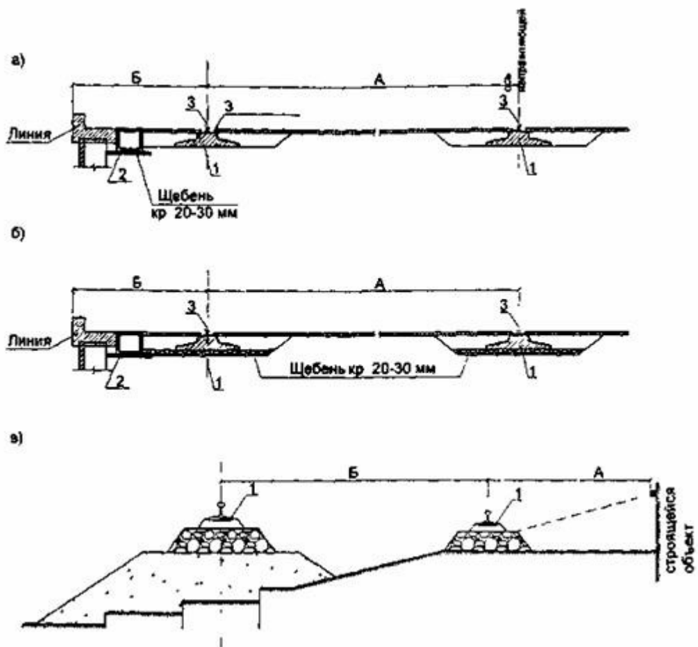
Рис. П.6.6. Поперечный профиль наземных крановых путей.
