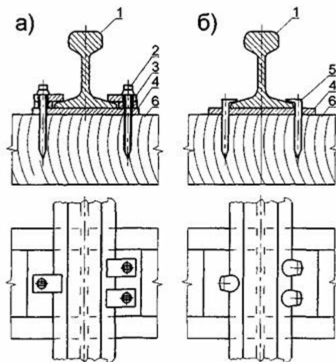
Рис. П.7.13. Прикрепление направляющих к полушпалам:
