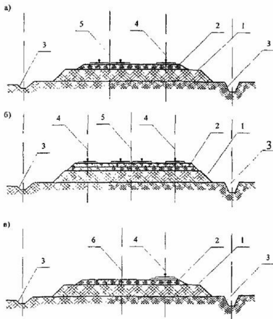
Рис. П.6.5. Поперечный профиль наземного кранового пути на общем земляном полотне
