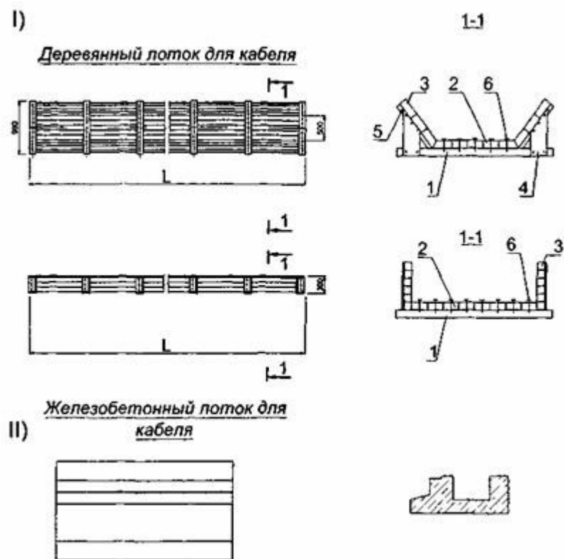
Рис. П.8.2. Лоток для укладки кабеля.
