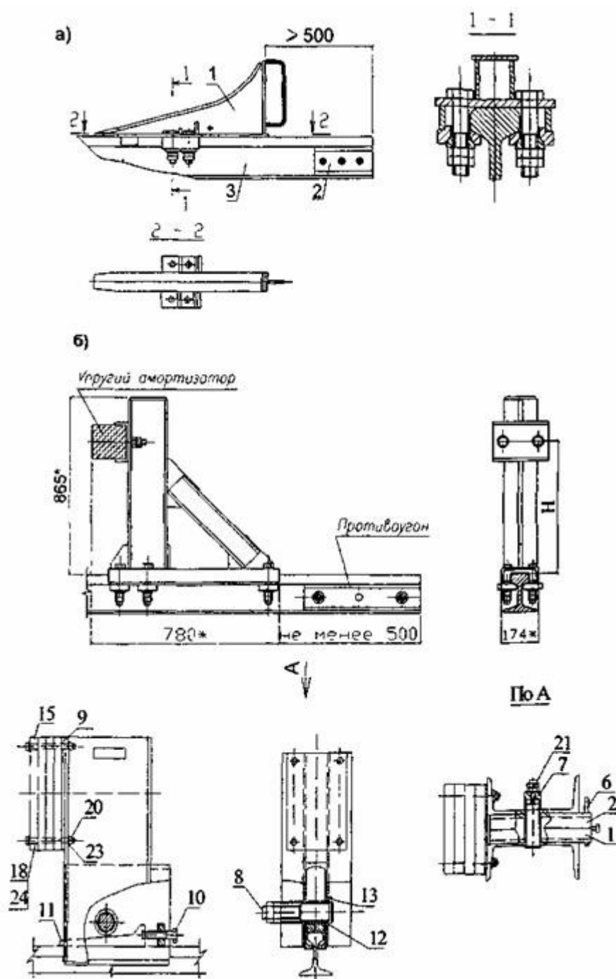
Рис. П.8.1. Тупиковые упоры
