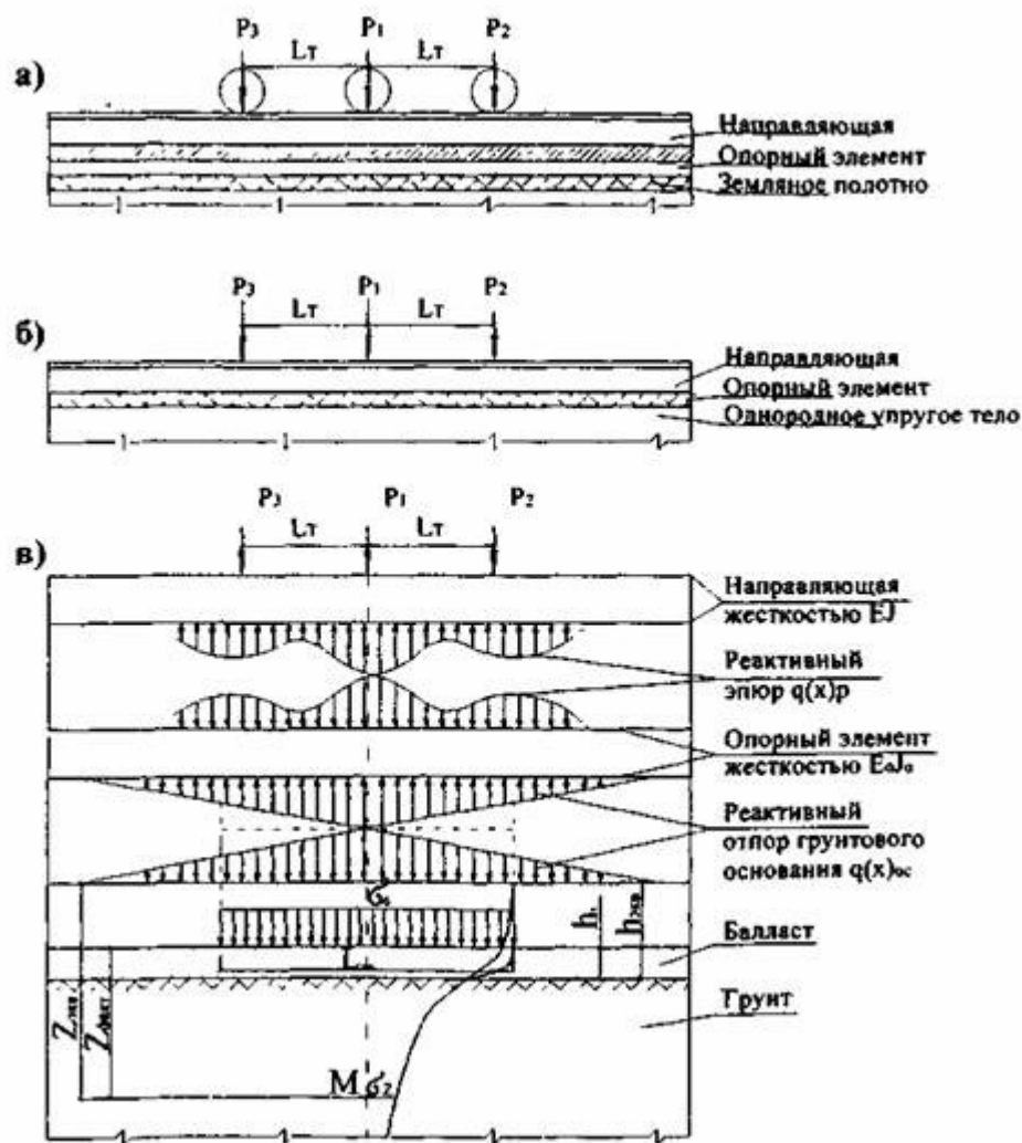
Рис. П.5.1. Расчетная схема наземного кранового пути
