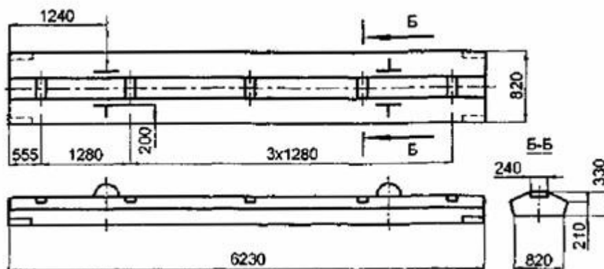
Рис. П.7.8. Железобетонная балка БПИ-62.8.3.
