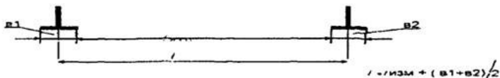
Рис. П.8.1. Измерение смещения оси балки кранового пути с продольной разбивочной оси
