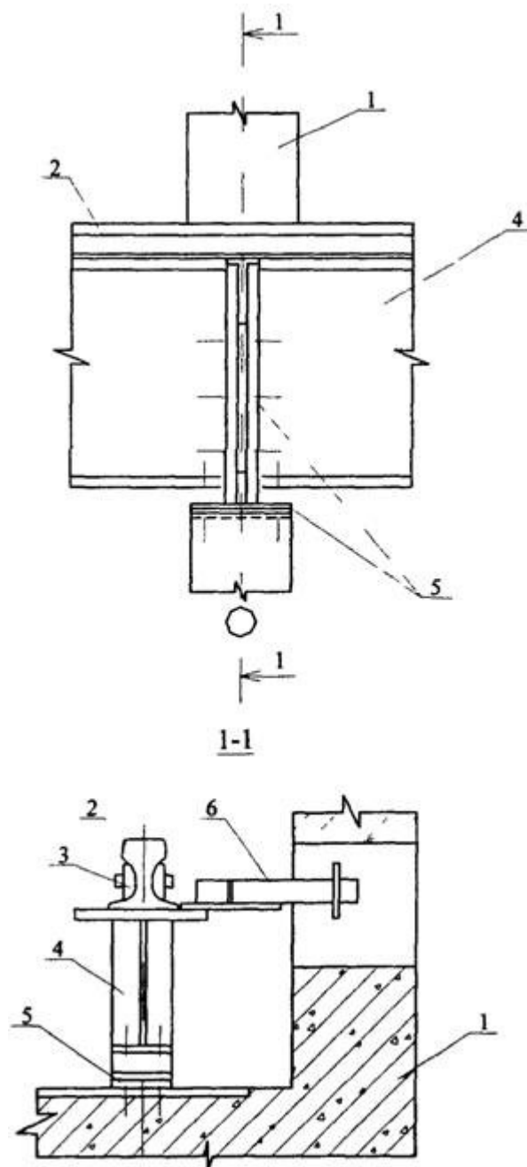
Рис. П.5.19. Узлы опирания и восстановление проектного положения балки кранового пути
