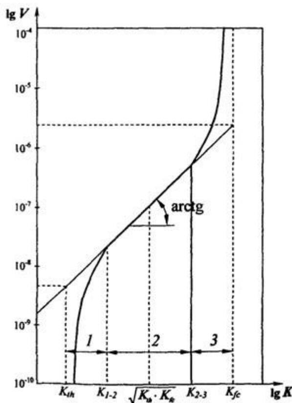
Рис. П.10.1. Типичная кинетическая диаграмма усталостного разрушения
