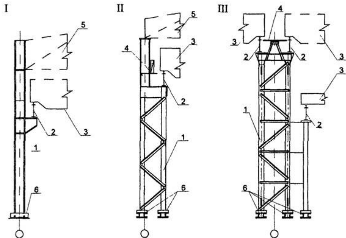
Рис. П.5.15. Типовые стальные опорные колонны надземных крановых путей
