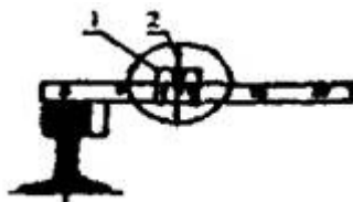
Рис. П.8.3. Определение расстояния от грани рельса до верхнего пояса балки кранового пути. Стальной угольник устанавливается по уровню
