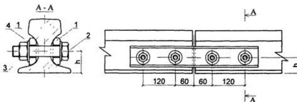
Рис. П.5.4. Разъемное стыковое крепление для направляющих типа КР
