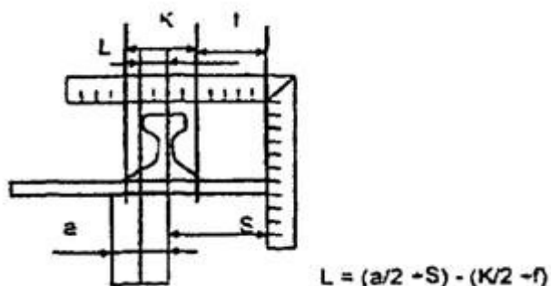
Рис. П.8.2. Замеры отклонения между осями соседних путей
