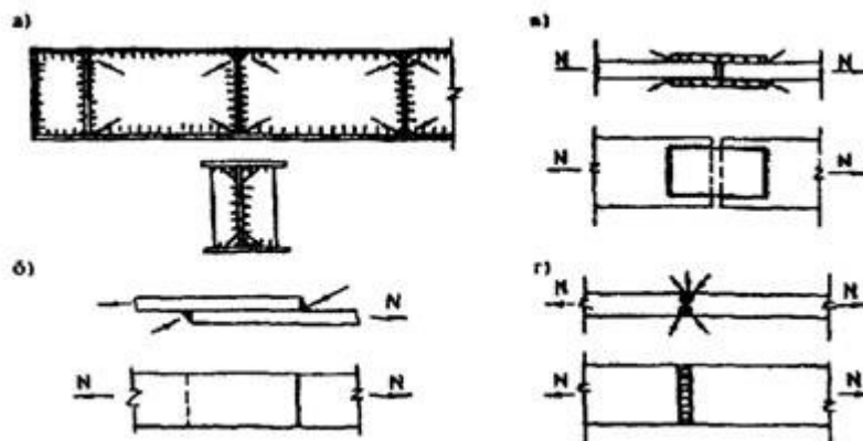
Рис. П.7.2. Места зарождения усталостных трещин в сварных соединениях элементов стальных конструкций кранового пути
