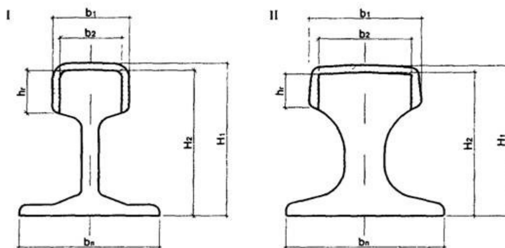
Рис. П.5.1. Поперечный профиль направляющих
