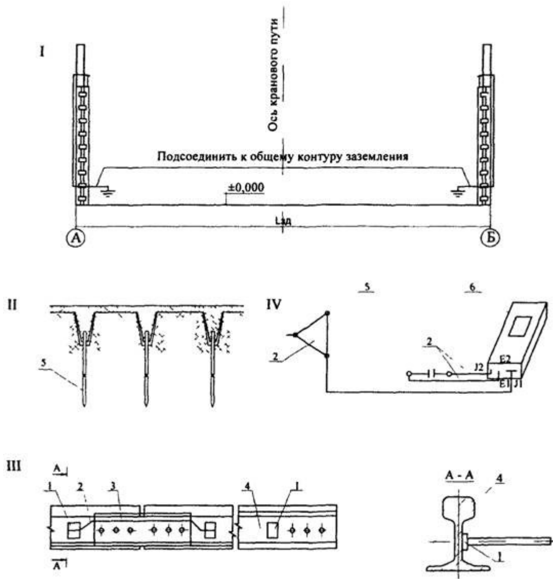
Рис. П.5.22. Система заземления надземных крановых путей.
