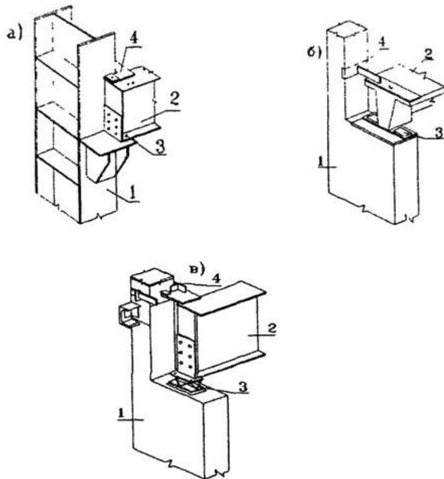
Рис. П.5.18. Узлы опирания балок кранового пути на колоннах
