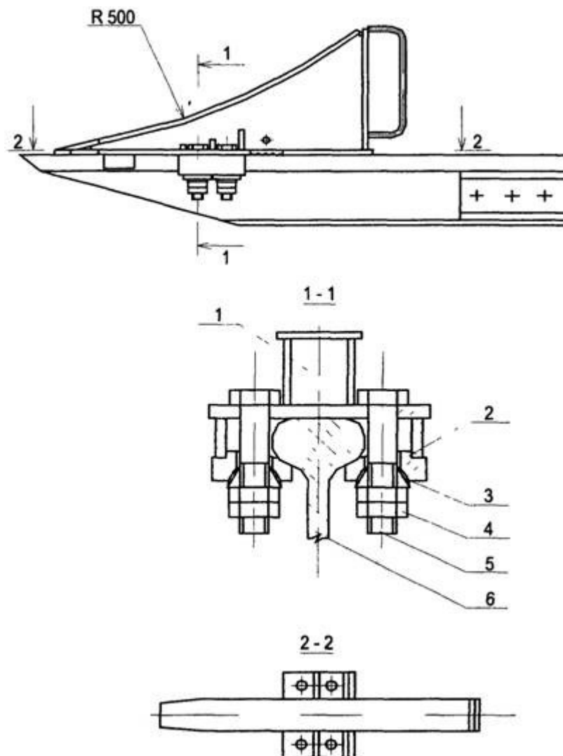
Рис. П.5.21. Тупиковый упор безударного типа
