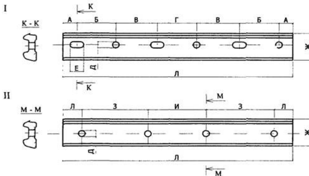
Рис. П.5.3. Стыковые двухголовые накладки для направляющих типа Р
