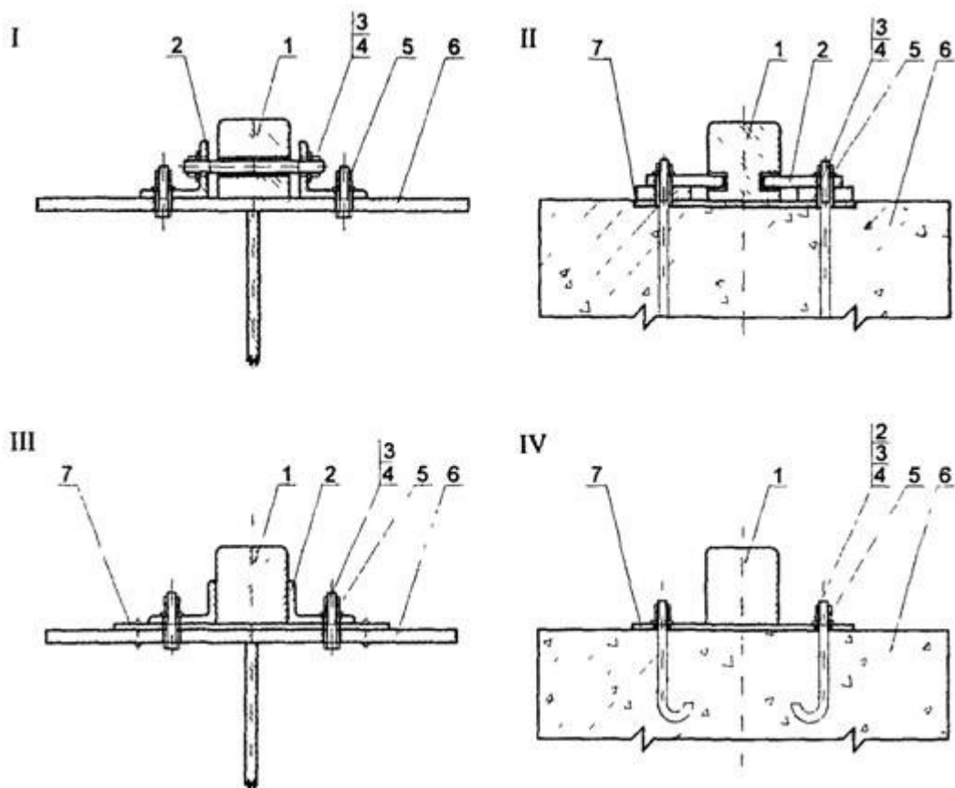
Рис. П.5.9. Промежуточные скрепления для крепления направляющей - стального горячекатаного квадрата к стальной и железобетонной балке кранового пути
