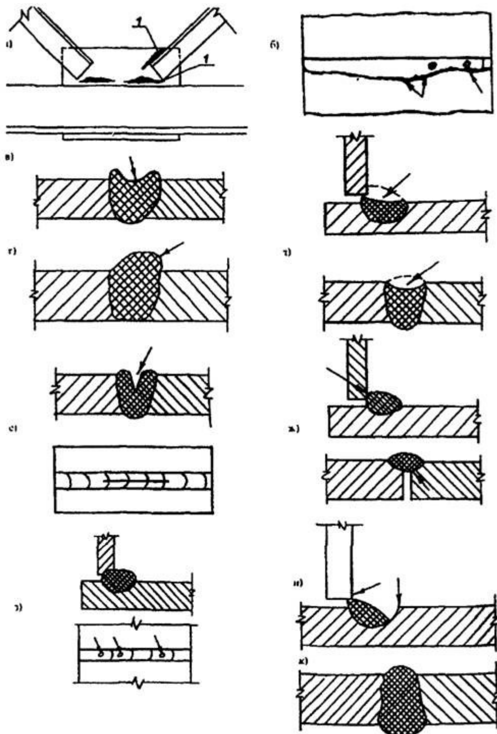
Рис. П.7.1. Дефекты повреждения сварных соединений стальных элементов и конструкций кранового пути
