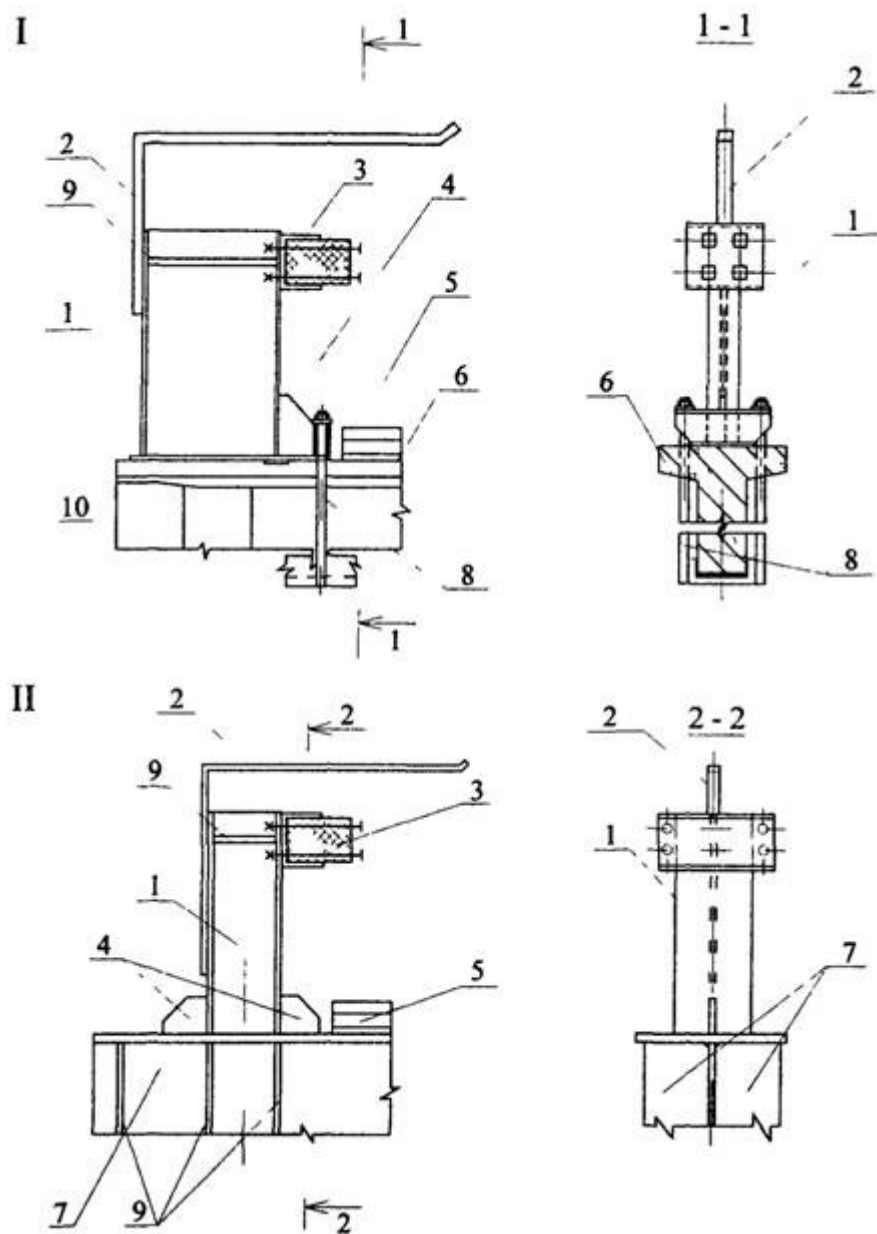
Рис. П.5.20. Тупиковый упор ударного типа на железобетонной (I) и металлической (II) балке кранового пути
