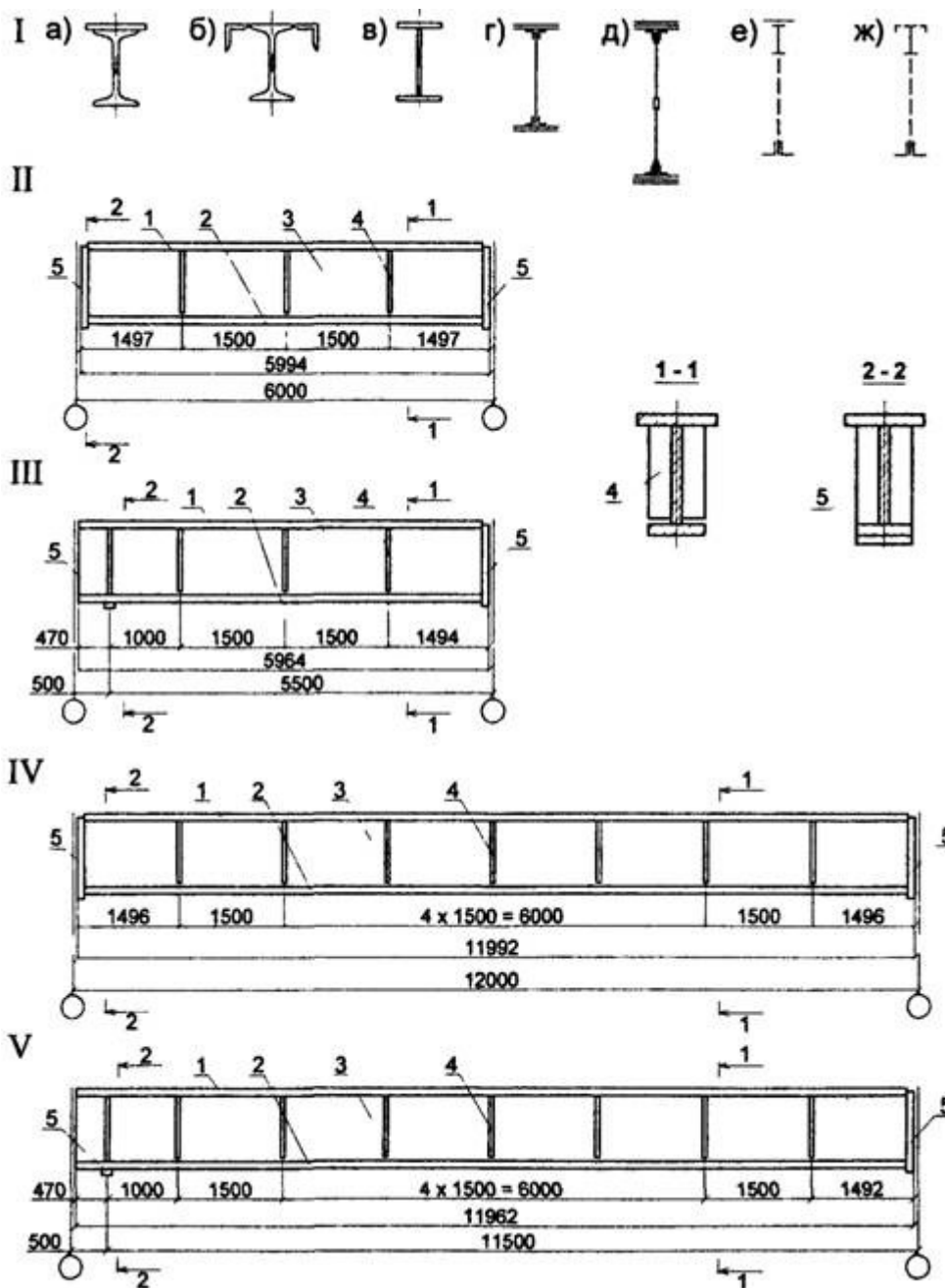
Рис. П.5.14. Сечения (I) и схемы (II) стальных балок кранового пути
