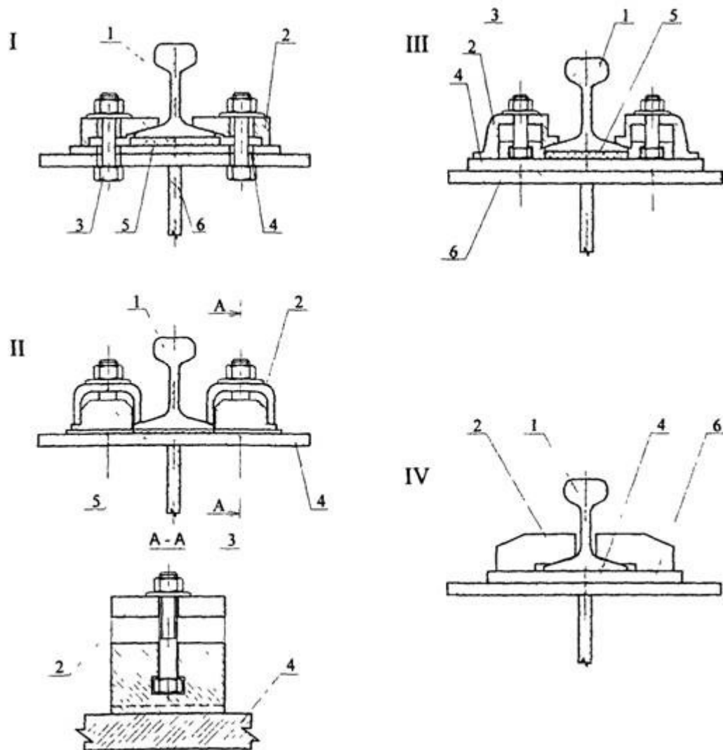
Рис. П.5.7. Промежуточные крепления для прикрепления направляющих к стальной балке кранового пути
