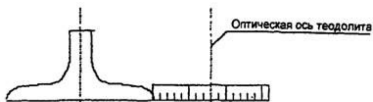
Рис. П.8.1. Измерение смещения оси балки кранового пути с продольной разбивочной оси
