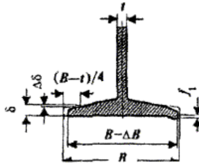
Рис. Схема проведения измерений величин износа и отгиба полки монорельса при проведении его дефектации.
