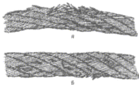
Рис. 3. Обрывы проволок в зоне уравнительного блика:
