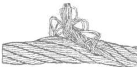
Рис. 11. Выдавливание сердечника
