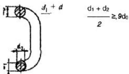
Рис 2. Уменьшение диаметра сечения звена цепи:
