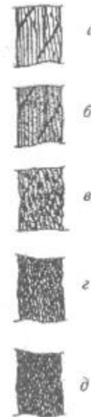
Рис. 6. Поверхностная коррозия проволок каната крестовой свивки:
