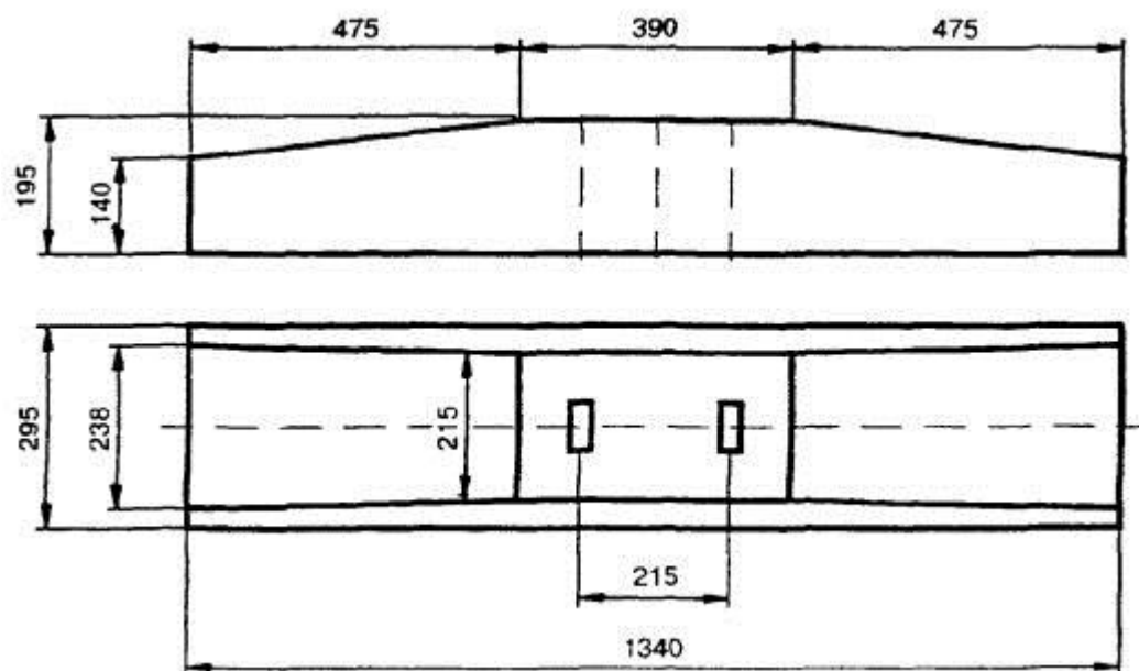
Б3. Железобетонная балка типа БРП-62.8.3
