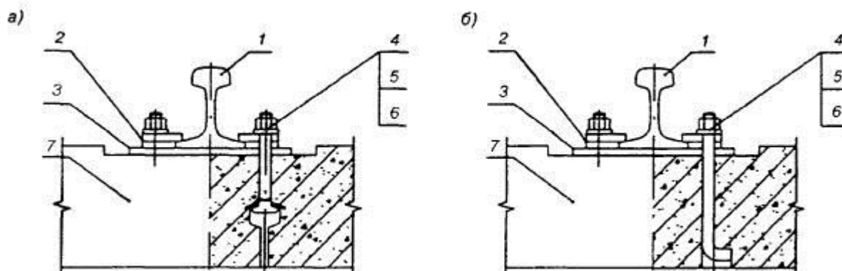
а - закладной болт по ГОСТ 16017 ; б - нестандартный анкерный закладной болт
