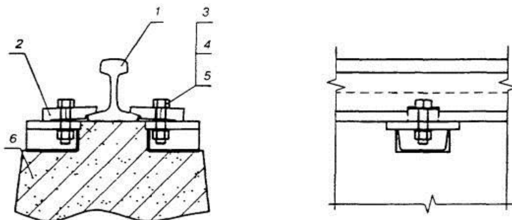
1 - рельс; 2 - прижим; 3 - закладной болт; 4 - гайка; 5 - шайба пружинная; 6 - железобетонный опорный элемент (балка)
