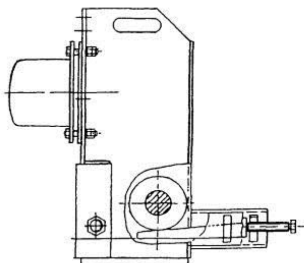
б) ударного типа
