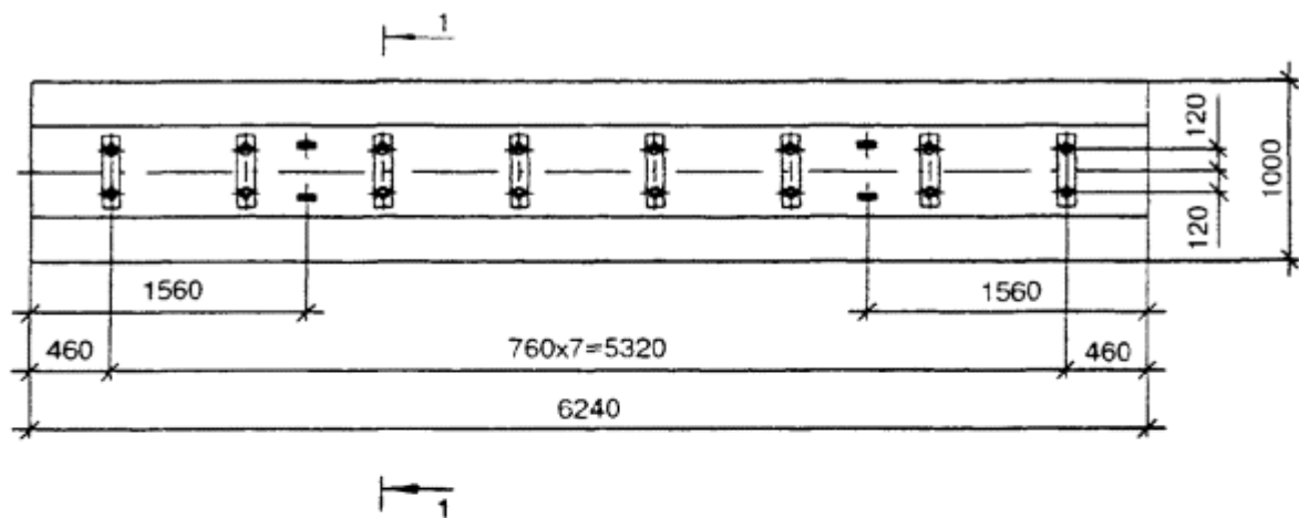
Б5. Железобетонная балка типа БРК-6.24-04
