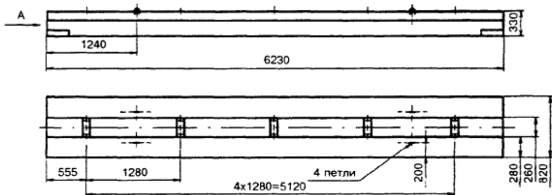
Б3. Железобетонная балка типа БРП-62.8.3
