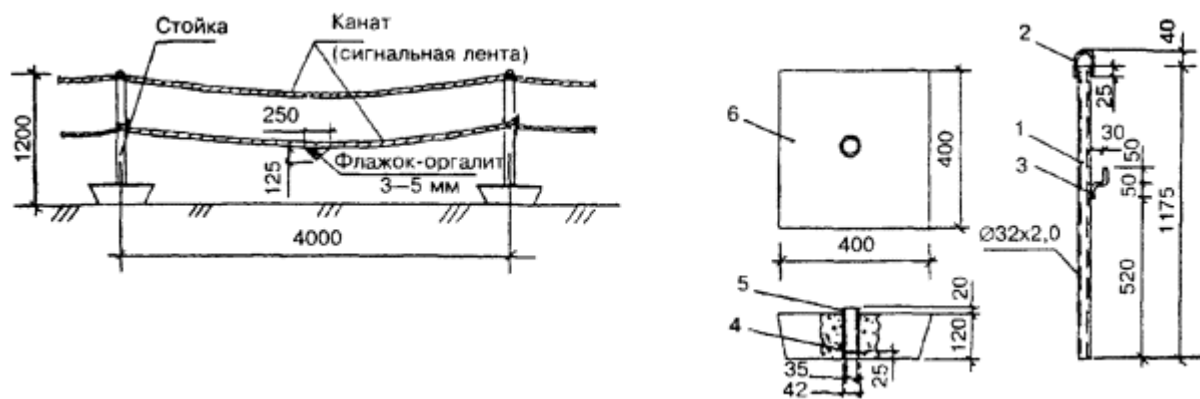
1 - стойка; 2 - скоба; 3 - полускоба; 4 - анкер; 5 - гильза; 6 - опора
