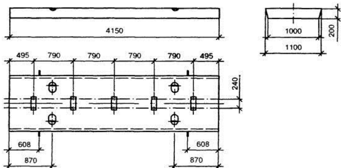
Б5. Железобетонная балка типа БРК-6.24-04
