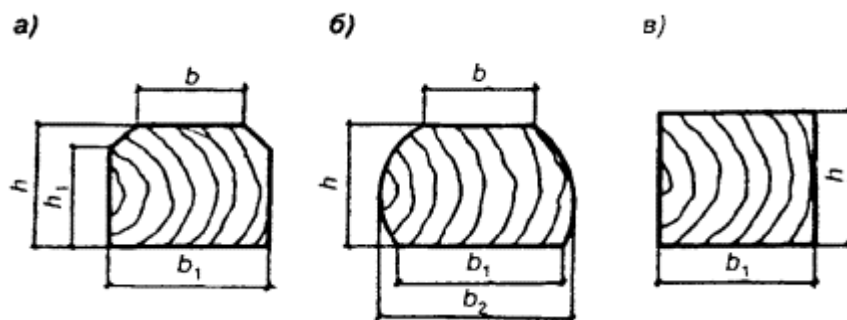
Поперечное сечение деревянных полушпал
